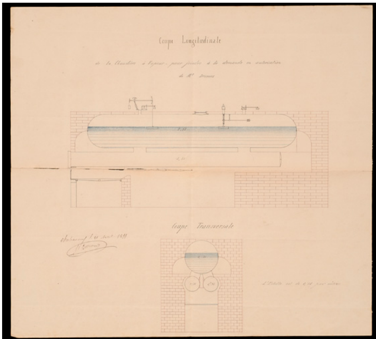
Moulin à vent et à vapeur de Prosper Desnoës. Coupe longitudinale de la chaudière à vapeur. Signé Desnoës à Châteauneuf le 21 avril 1855. (ADML - 50 M 22)
