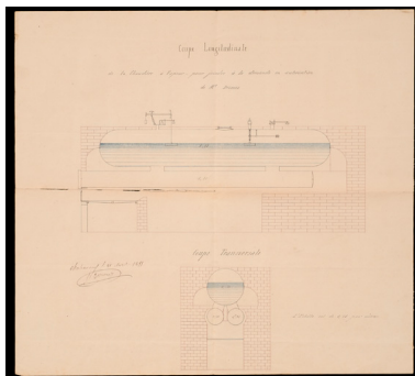
Moulin à vent et à vapeur de Prosper Desnoës. Coupe longitudinale de la chaudière à vapeur. Signé Desnoës à Châteauneuf le 21 avril 1855. (ADML - 50 M 22) Repro. Bruno Rousseau, Autr. Prosper Desnoës IVR52_20074900237NUCA
