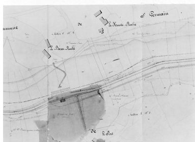
Projet (réalisé) de barrage et d'écluse du Port. Plan d'ensemble extrait du plan parcellaire des bords de la Mayenne à canaliser entre Sacé et le pont de Montgiroux. Autr. Charles Dupuy, Repro. François Lasa IVR52_20025300263X
