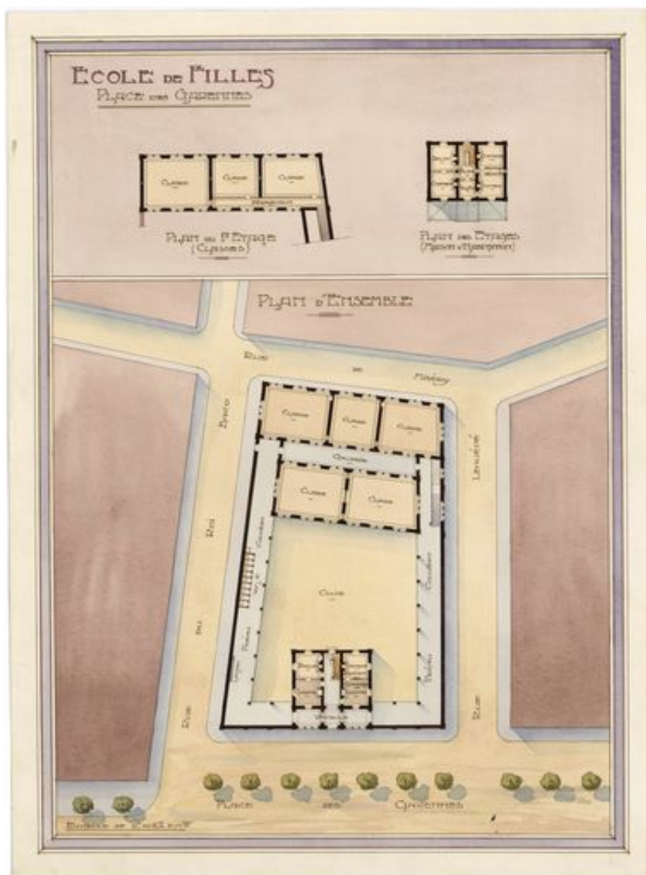
Plan de l'école des filles, 1878.
