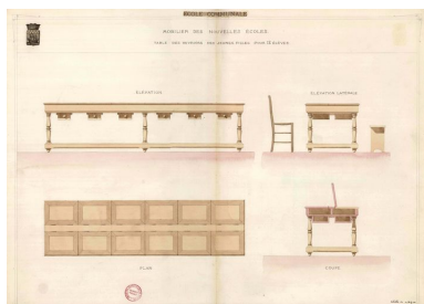
Plan des ouvroirs pour jeunes filles, 1878. Phot. Patrick (reproduction) Jean IVR52_20124400455NUCA
