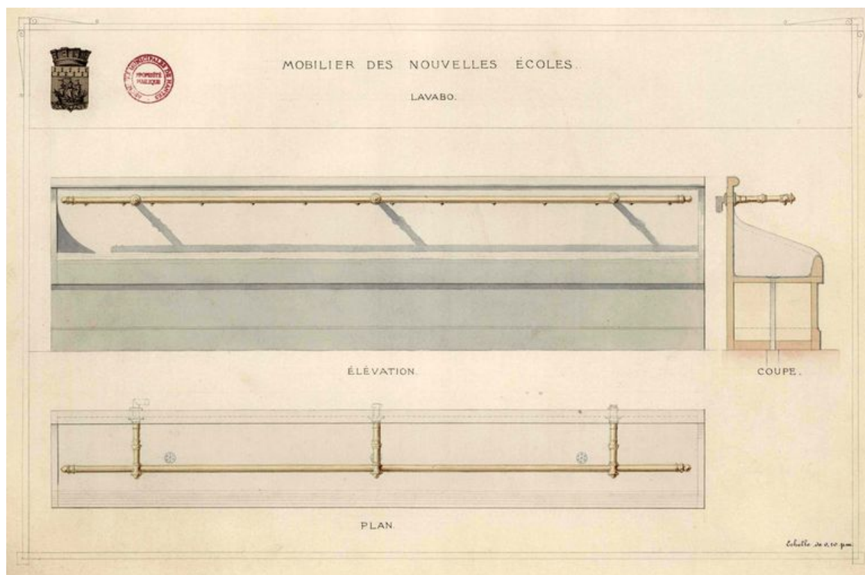
Plan des lavabos, 1878.
