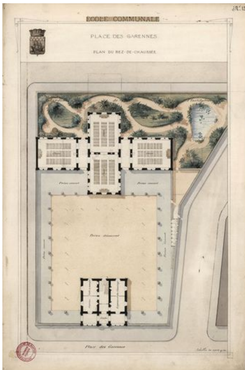
Plan de l'école des garçons, 1878.
