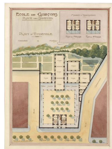
Plan de l'école des garçons avec des classes supplémentaires, fin du XIXe siècle. Phot. Patrick (reproduction) Jean IVR52_20124400401NUCA
