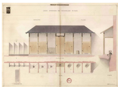
Plan des toilettes, 1878. Phot. Patrick (reproduction) Jean IVR52_20124400474NUCA
