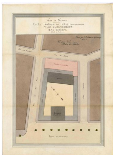
Projet d'agrandissement de l'école des filles, 1902. Phot. Patrick (reproduction) Jean IVR52_20124400440NUCA
