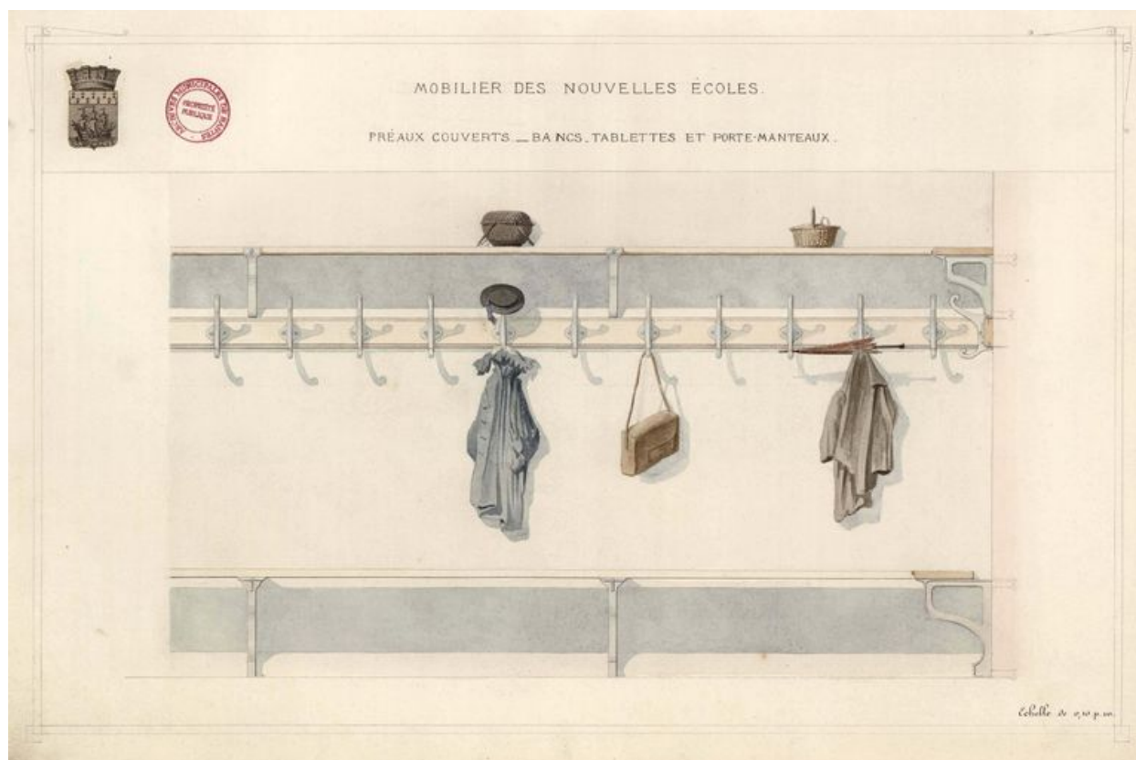
Plan des tablettes et des porte-manteaux, 1878.
