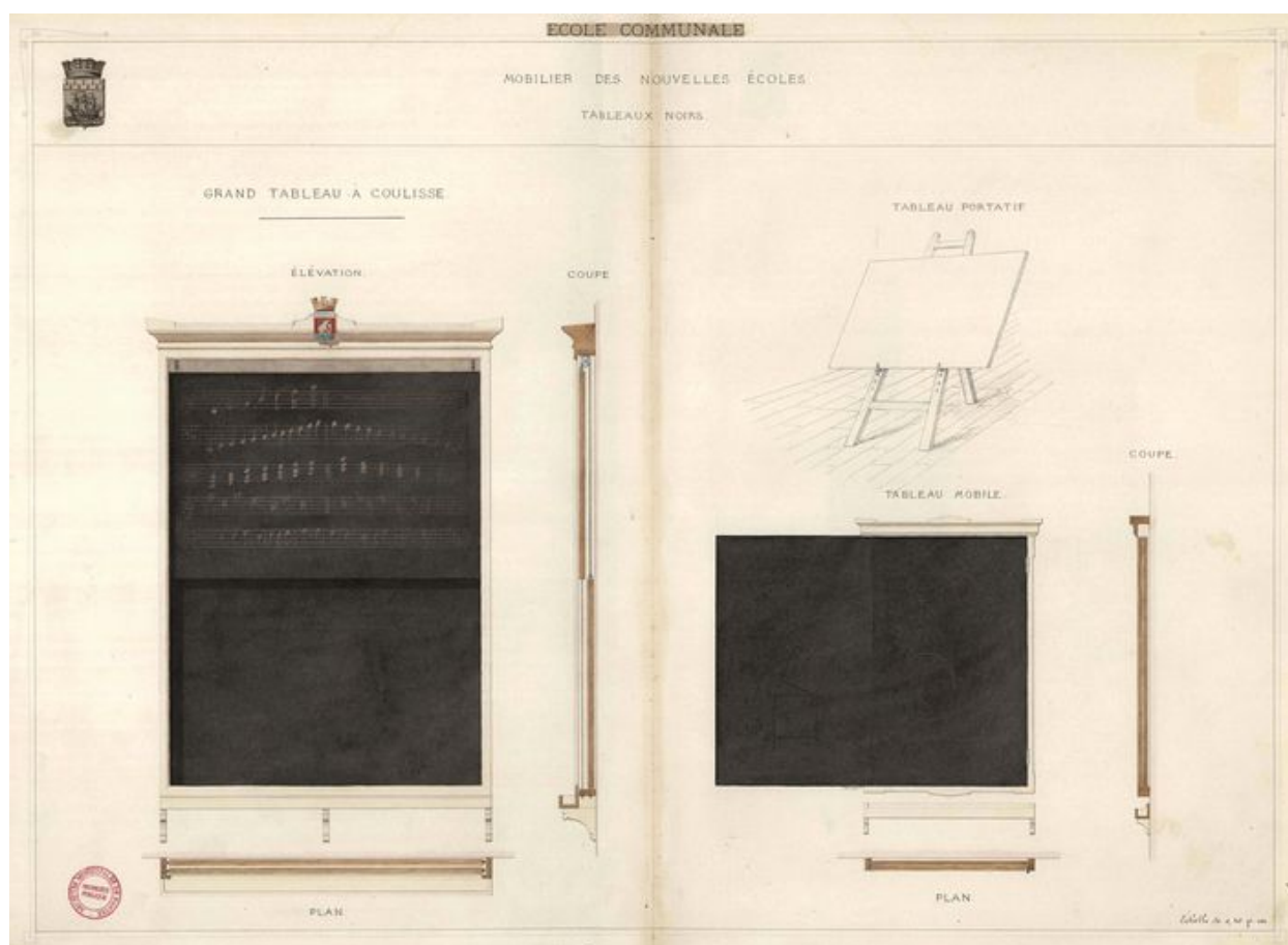
Plan des tableaux noirs, 1878.
