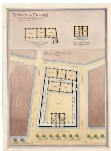
Plan de l'école des filles, 1878. Phot. Patrick (reproduction) Jean IVR52_20124400427NUCA
