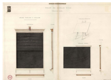
Plan des tableaux noirs, 1878. Phot. Patrick (reproduction) Jean IVR52_20124400449NUCA
