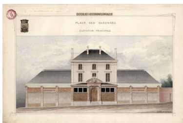
Elévation du porche et du bâtiment d'entrée de l'école des garçons, 1878. Phot. Patrick (reproduction) Jean IVR52_20124400406NUCA
