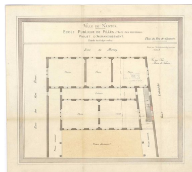
Projet d'agrandissement de l'école des filles, 1902. Phot. Patrick (reproduction) Jean IVR52_20124400435NUCA
