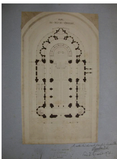
Projet n° 1 pour la construction de l'église du Sacré-Cœur de Paris. Phot. Françoise (reproduction) Lelièvre IVR52_20074400020NUCA
