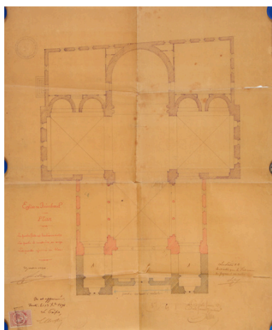
Plan d'ensemble en 1894 : le sanctuaire réalisé (hachures violettes), la nef à construire (hachures rouges), le massif antérieur restant à exécuter.
