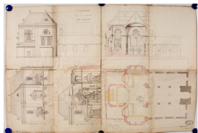
Premier projet de reconstruction, par Charpentier (architecte), 1870 (en jaune et en gris, le plan de l'église construite au XVIIIe siècle). Autr. Louis Charpentier, Phot. Denis (reproduction) Pillet IVR52_20044400155NUCA
