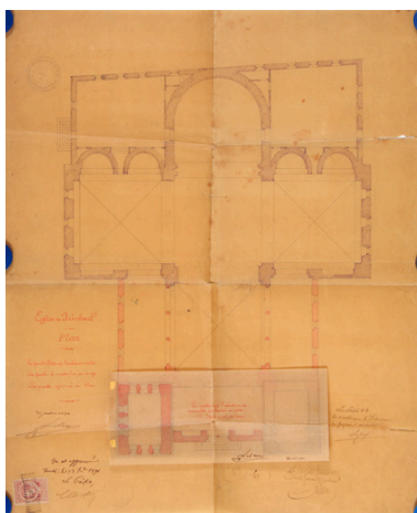
Plan d'ensemble (1894) avec retombe ajoutée le 26 août 1904 : plan du massif antérieur (à construire) modifié.
