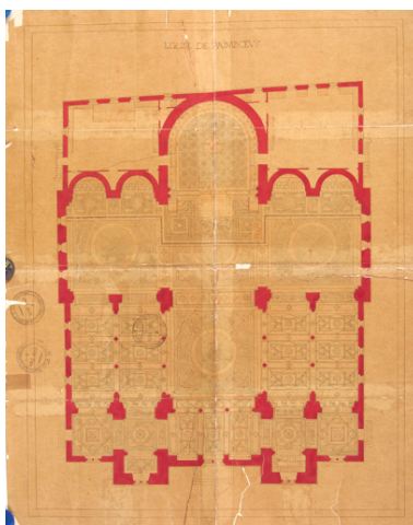
Plan d'ensemble avec pavements [1876] avant la suppression de deux bas-côtés. Autr. Ludovic Douillard, Phot. Denis (reproduction) Pillet IVR52_20044400154NUCA
