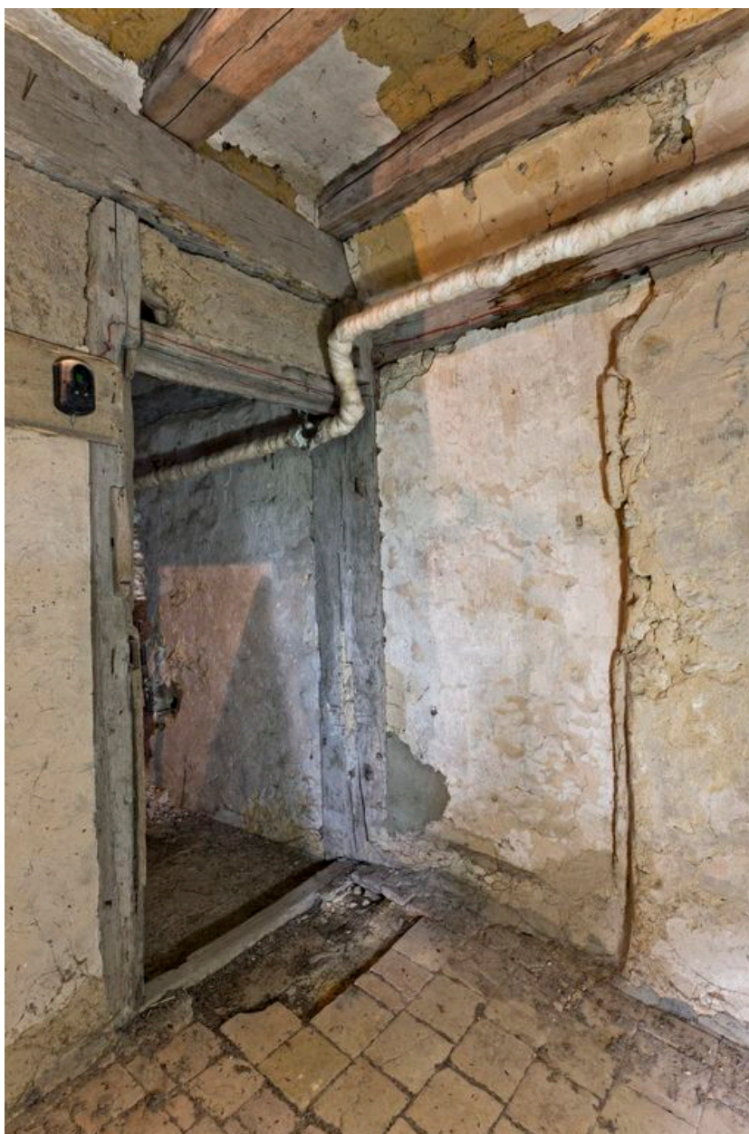
Pièce 3, porte d'accès depuis la pièce 2 et ancienne porte (?) dans l'élévation postérieure
