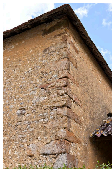
mur-pignon gauche de la grange-étable-fenil Phot. Yves Guillotin IVR52_20137200519NUCA
