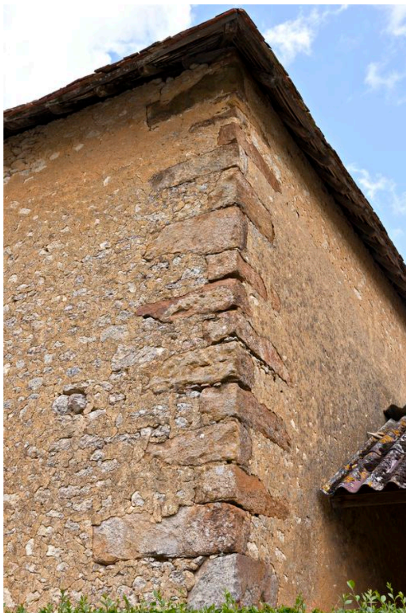
Détail de la chaîne d'angle antérieure droite de la grange-étable-fenil.
