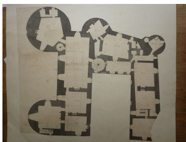
Plan du 1er étage vers 1750-1770, par Boulard ? Autr. Boulard (architecte), Phot. Christine (reproduction) Toulhier IVR52_20147201212NUCA
