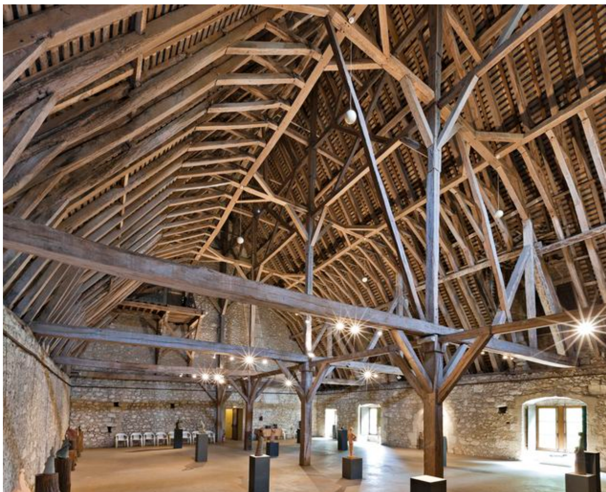
Charpente des greniers à blé en surcroît : charpente à pannes avec deux sous-faîtages.
