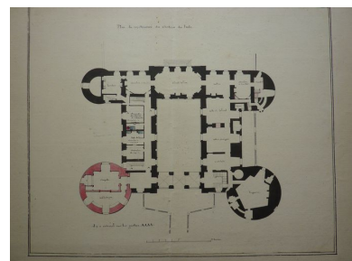
Plan du château du Lude selon Vincent Barré. Autr. Vincent (architecte) Barré, Phot. Christine (reproduction) Toulhier IVR52_20147201214NUCA
