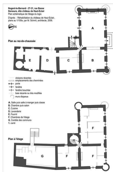
Plans schématiques du rez-de-chaussée et de l'étage carré du logis Dess. Julien Hardy IVR52_20137200041NUDA
