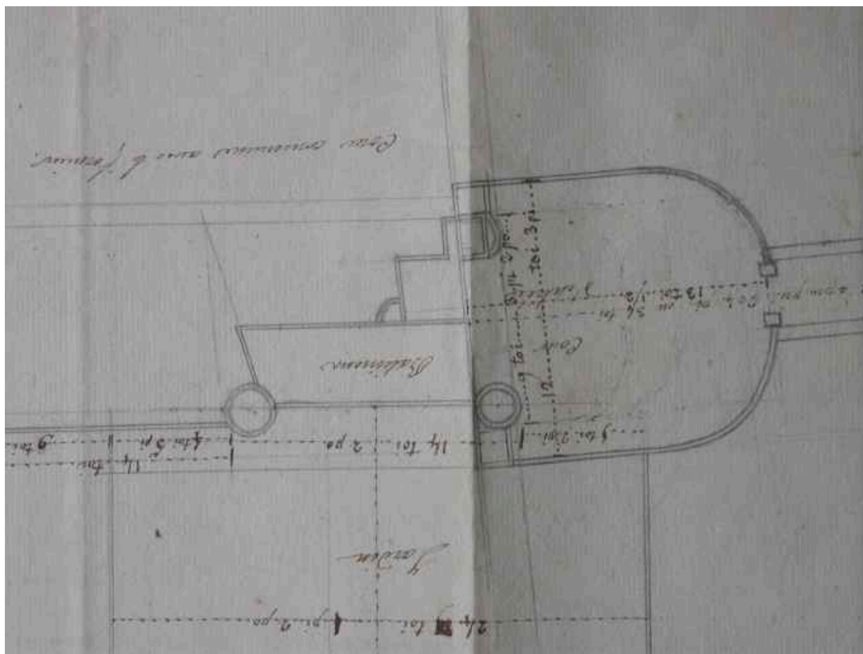
Plan coté du logis au XVIIIe siècle. Dessin au crayon, coté, n.d., échelle en ligne. (Collection particulière).
