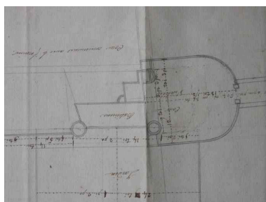
Plan coté du logis au XVIIIe siècle. Dessin au crayon, coté, n.d., échelle en ligne. (Collection particulière). Phot. Christine (reproduction) Toulhier IVR52_20057203959NUCA
