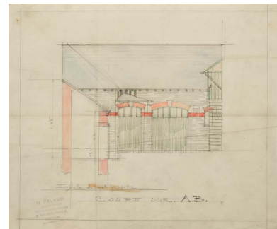
Propriété de M. Raout, construction d'une maison d'habitation. Coupe sur AB. Architecte : Henri Palausi. Non daté. Repro. Bruno Rousseau IVR52_20164900345NUCA
