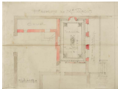
Propriété de M. Raout, construction d'une maison d'habitation. Architecte : Henri Palausi. Non daté. Repro. Bruno Rousseau IVR52_20164900344NUCA
