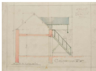
Propriété de M. Raout, construction d'une maison d'habitation. Architecte : Henri Palausi. Non daté.
