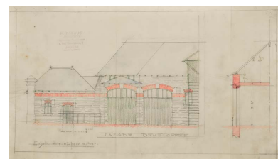
Propriété de M. Raout, construction d'une maison d'habitation. Façade développée. Architecte : Henri Palausi. Non daté.
