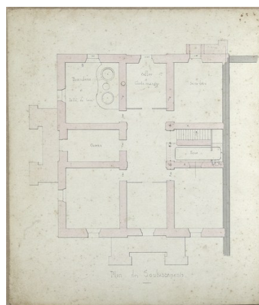
Plan du soubassement de la maison Phelippon par Léon Ballereau, en 1874. Autr. Léon Ballereau, Phot. Patrice (reproduction) Giraud IVR52_20088500898NUCA
