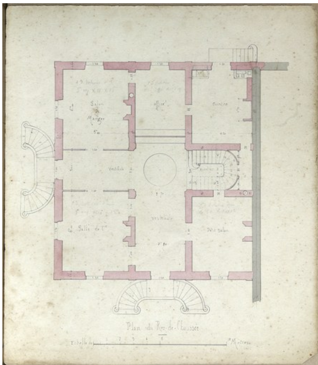
Plan du rez-de-chaussée par Léon Ballereau en 1874.
