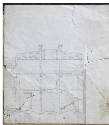
Coupe longitudinale Léon Ballereau en 1874. Autr. Léon Ballereau, Phot. Patrice (reproduction) Giraud IVR52_20088500899NUCA
