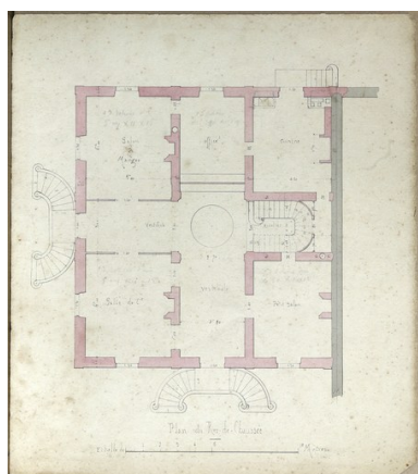
Plan du rez-de-chaussée par Léon Ballereau en 1874. Autr. Léon Ballereau, Phot. Patrice (reproduction) Giraud IVR52_20088500897NUCA
