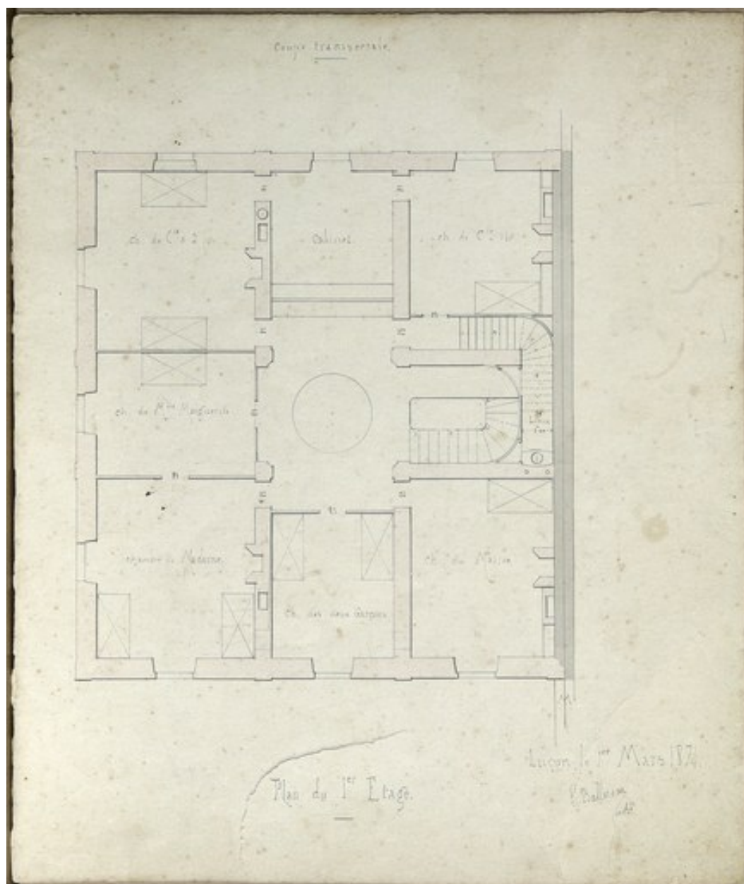
Plan du premier étage par Léon Ballereau en 1874.
