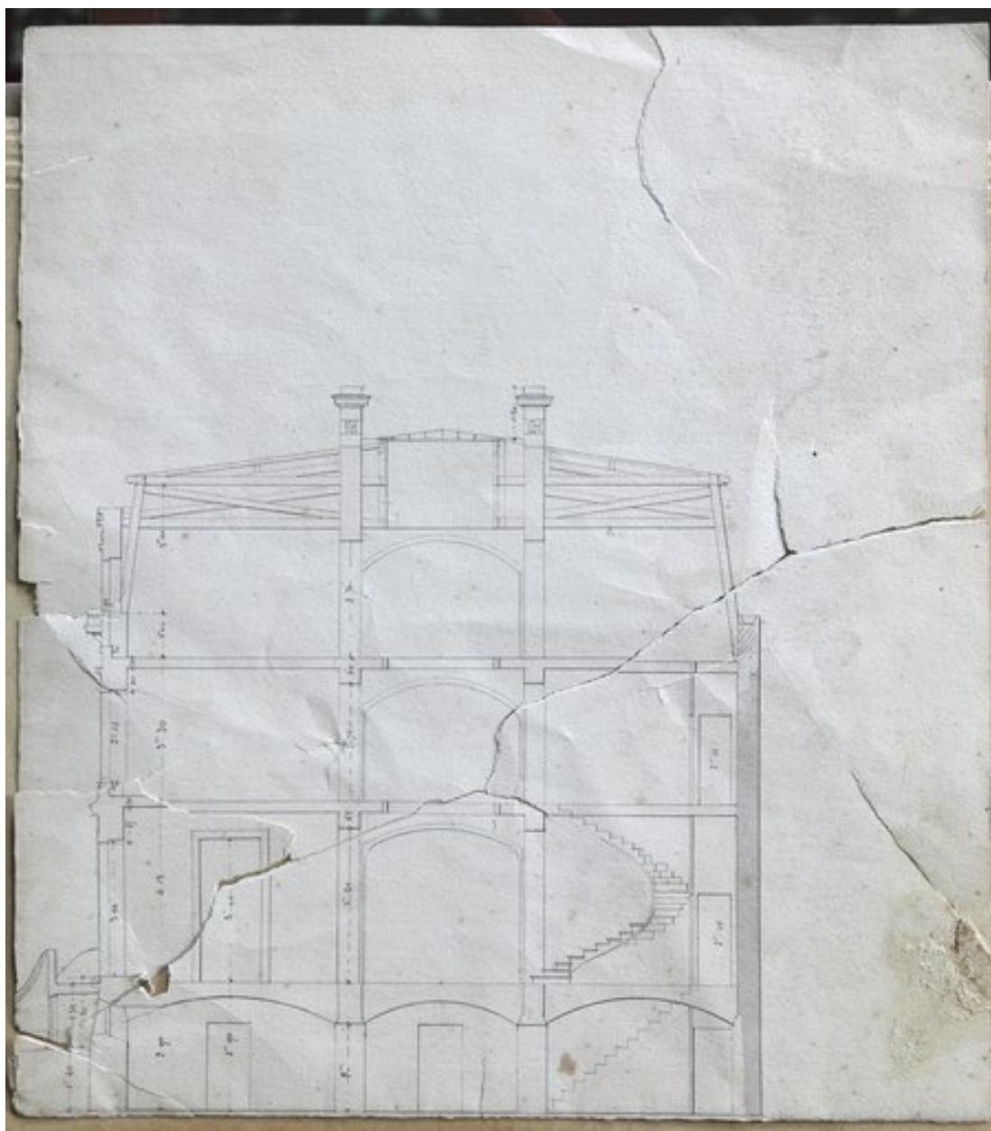
Coupe longitudinale Léon Ballereau en 1874.
