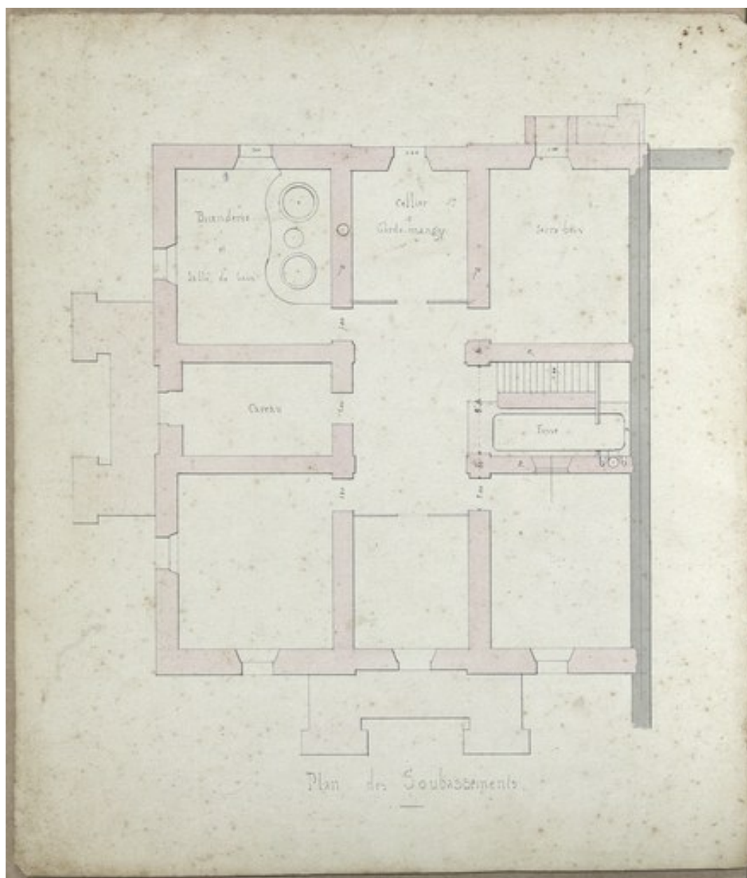
Plan du soubassement de la maison Phelippon par Léon Ballereau, en 1874.
