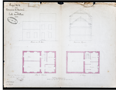
Les plans de l'ancienne école de filles, 1851. Phot. Pierre-Bernard Fourny, Phot. Nourry-Blottin IVR52_20187200632NUCA
