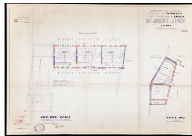
Le projet d'agrandissement de l'école de filles (non réalisé), par R. Cagnault, 1937, plans du premier étage. Phot. Pierre-Bernard Fourny, Phot. Raoul Cagnault IVR52_20187200633NUCA
