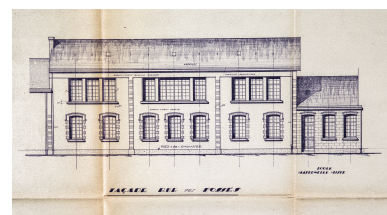
Le projet d'agrandissement de l'école de filles (non réalisé), par R. Cagnault, 1937, plans des classes, détail.
