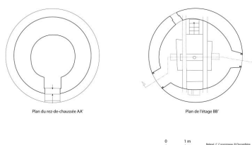
Plans du rez-de-chaussée et de l'étage du moulin de Drézeux. Dessin, C. Cussonneau, R. Durandière. Dess. Christian Cussonneau, Dess. Ronan Durandière IVR52_20104400568NUDA
