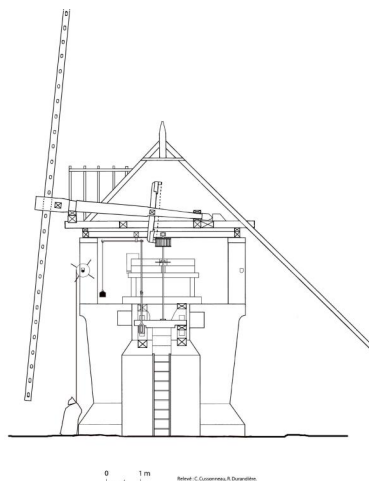
Reconstitution hypothétique du moulin en coupe. Deuxième trempure à trois leviers, circulation verticale intérieure. Autr. Christian Cussonneau, Autr. Ronan Durandière, Phot. Christian (reproduction) Cussonneau IVR52_20094401686NUCA
