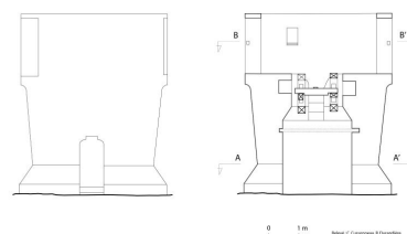
Élévation et coupe en AB du moulin de Drézeux. Dess. Christian Cussonneau, Dess. Ronan Durandière IVR52_20104400567NUDA
