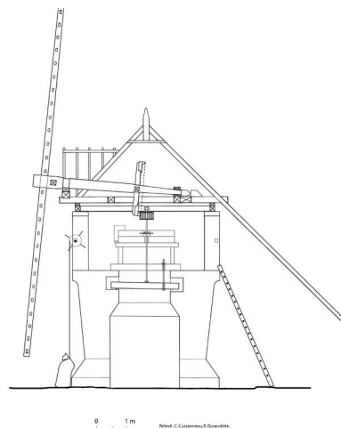
Reconstitution hypothétique du moulin en coupe. Trempure primitive à un seul levier et vis de réglage. Courant du XIVe siècle. Phot. Christian (reproduction) Cussonneau, Autr. Christian Cussonneau, Phot. Ronan Durandière IVR52_20094401683NUCA
