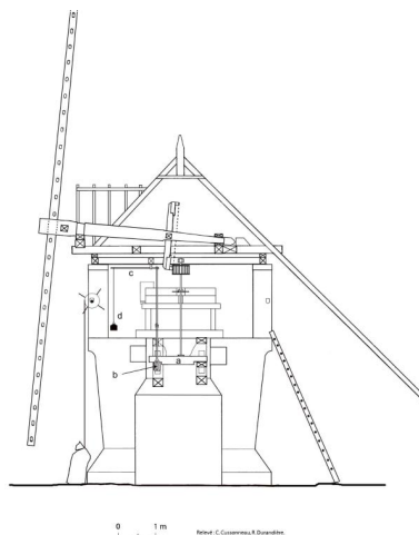
Deuxième trempure à trois leviers, circulation verticale extérieure (a : 3e levier (palier) ; b : 2e levier ; c : 3e levier ; d : contrepoids). Fin XIVe siècle jusqu'au XVIIe siècle (?). Autr. Christian Cussonneau, Phot. Christian (reproduction) Cussonneau, Autr. Ronan Durandière IVR52_20094401684NUCA
