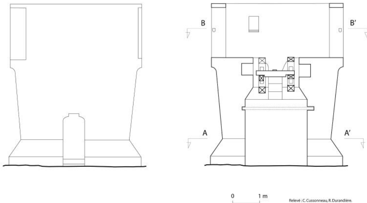
Élévation et coupe en AB du moulin de Drézeux.
