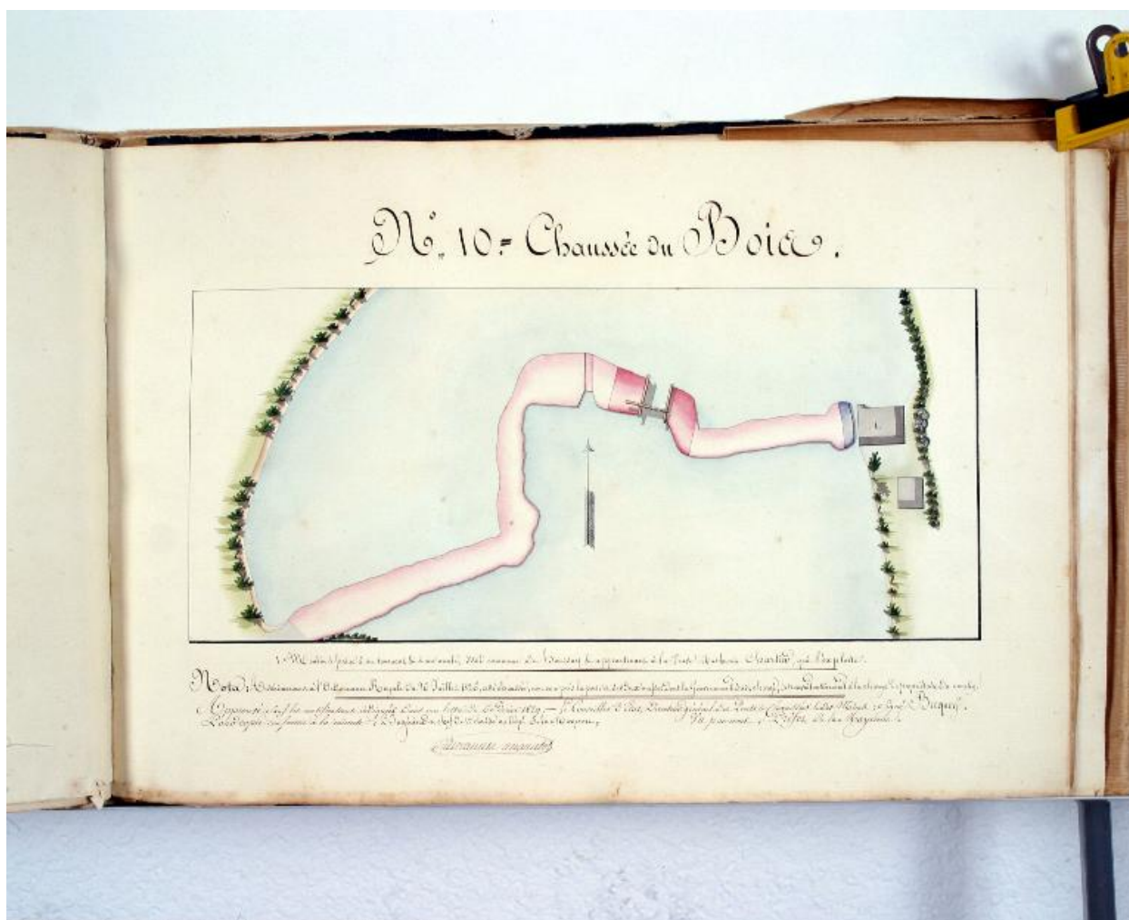
Planche N° 10 du recueil des plans des barrages de la partie navigable de la Mayenne. Plan d'ensemble du site du Bois avant la canalisation de la rivière : barrage, porte marinière, moulin à farine.
