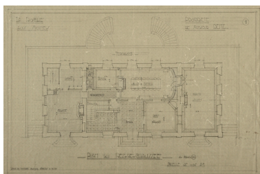
Propriété de M. Benz. Plan du rez-de-chaussée. Architecte : Ernest Bricard. 1926. Repro. Bruno Rousseau IVR52_20164901111NUCA
