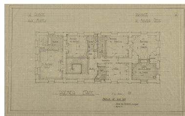
Propriété de M. Benz. Plan du 1er étage. Architecte : Ernest Bricard. 1926. Repro. Bruno Rousseau IVR52_20164901112NUCA
