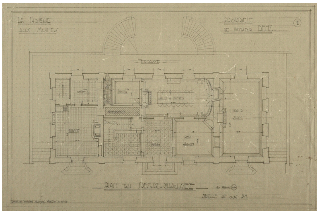
Propriété de M. Benz. Plan du rez-de-chaussée. Architecte : Ernest Bricard. 1926.
