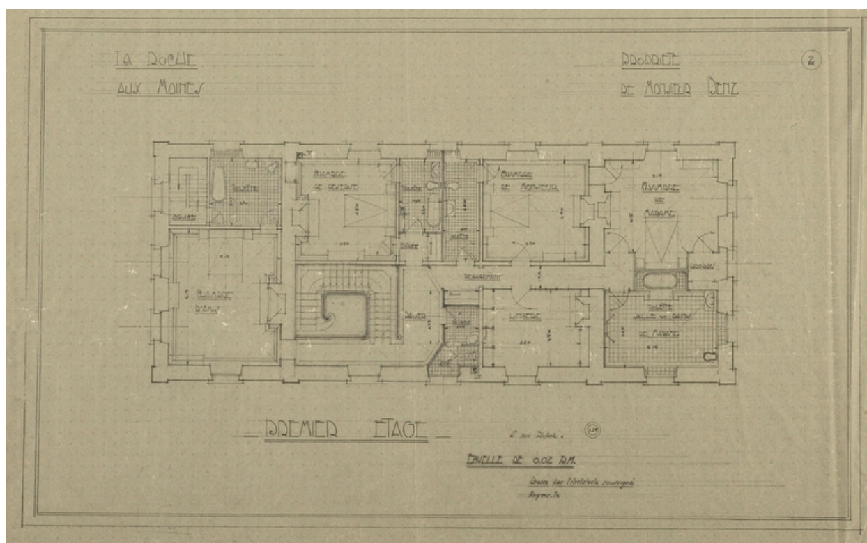
Propriété de M. Benz. Plan du 1er étage. Architecte : Ernest Bricard. 1926.
