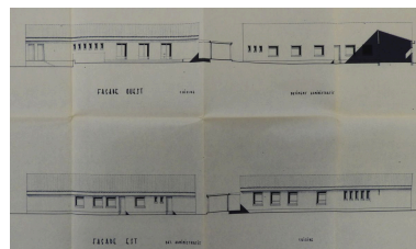
Projet en 1964 : élévations du bâtiment administratif et du réfectoire. Phot. Yannis (reproduction) Suire IVR52_20198500924NUCA
