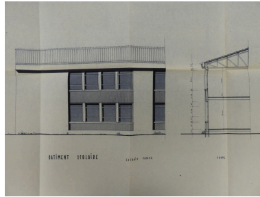
Projet de collège en 1964 : détail de façade et coupe du bâtiment ouest. Phot. Yannis (reproduction) Suire IVR52_20198500934NUCA
