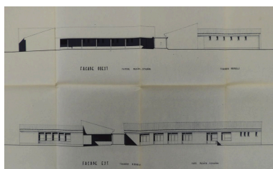
Projet de collège en 1964 : élévations de la salle d'études et de la salle de technologie. Phot. Yannis (reproduction) Suire IVR52_20198500925NUCA
