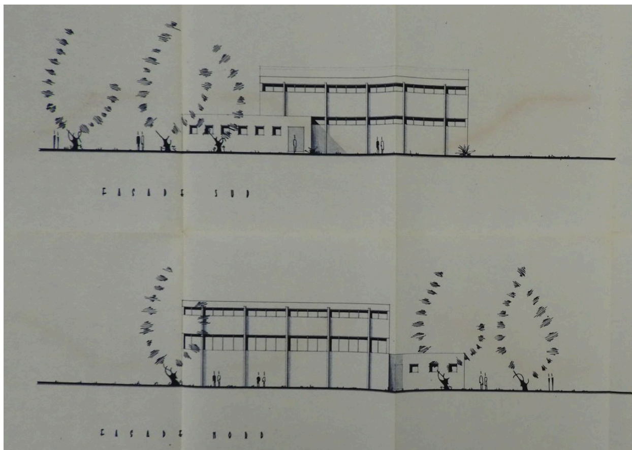
Projet de collège en 1964 : élévations du gymnase.
