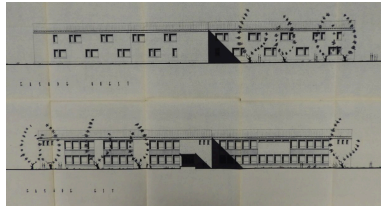
Projet de collège en 1964 : élévations du bâtiment ouest. Phot. Yannis (reproduction) Suire IVR52_20198500932NUCA
