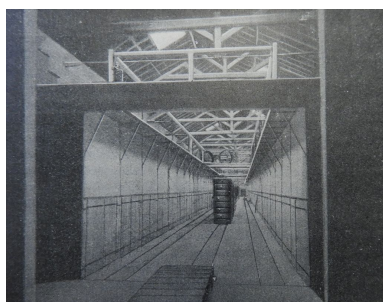
Usine de vaseline de L'Île-d'Elle : la salle de filtration en 1920 ; au centre, une batterie d'éléments prêts à être placés dans une chambre. Phot. Yannis (reproduction) Suire IVR52_20198501001NUCA
