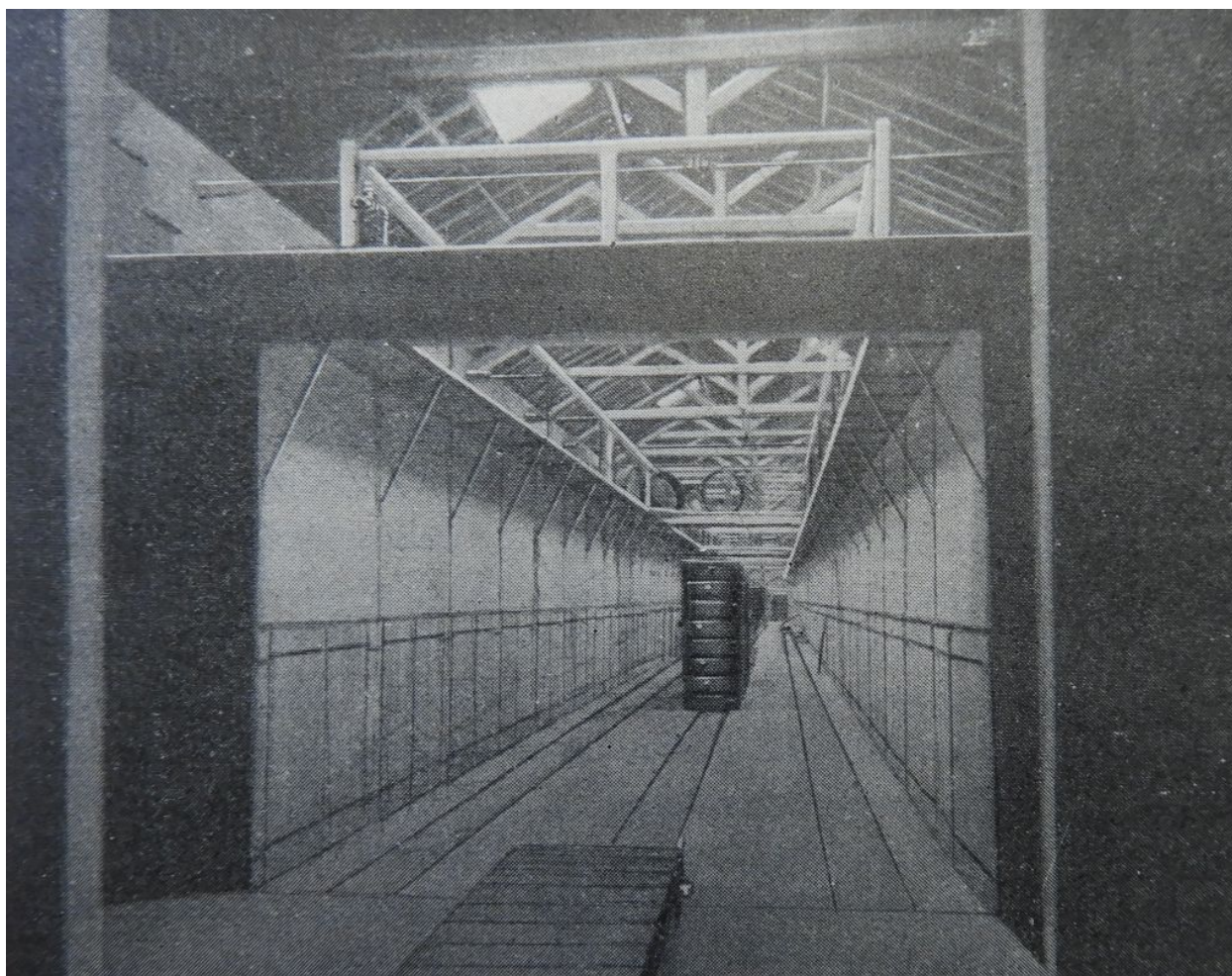
Usine de vaseline de L'Île-d'Elle : la salle de filtration en 1920 ; au centre, une batterie d'éléments prêts à être placés dans une chambre.
