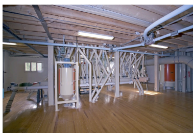
Minoterie, premier étage : le mélangeur Sangati et les conduites à aspiration. Phot. François Lasa IVR52_20075300791NUCA
