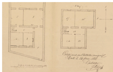
Plan de l'école communale de filles de la commune de Maillé, 24 février 1882 : détail, plans du rez-de-chaussée et de l'étage.
