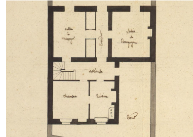
Plan de la maison du curé Gaudineau, par Auguste Garnereau, 10 février 1849 : détail, plan au rez-de-chaussée.
