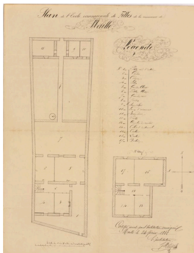
Plan de l'école communale de filles de la commune de Maillé, 24 février 1882.
