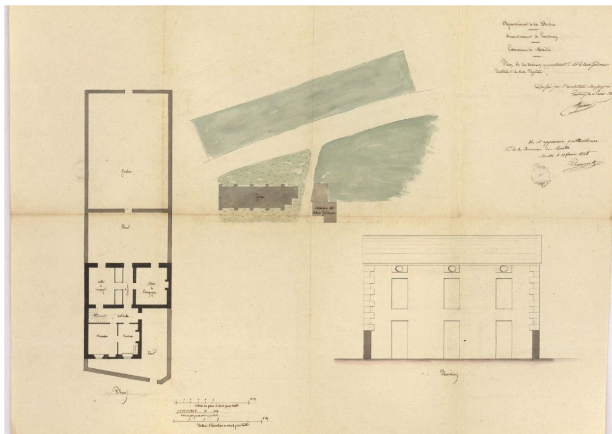
Plan de la maison du curé Gaudineau, par Auguste Garnereau, 10 février 1849.
