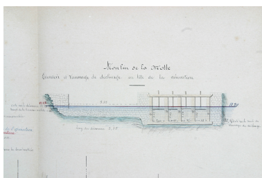
Dessin des ouvrages régulateurs établi à l'occasion du projet de règlement du moulin en 1880. Autr. J. Legras, Phot. François Lasa IVR52_20035302306NUCA
