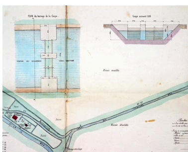
Le barrage de la Coupe (détail d'un plan de Dabin, le 2 juillet 1860). Autr. Dabin, Phot. Christophe (reproduction) Yvernoiseau IVR52_19998500375XA
