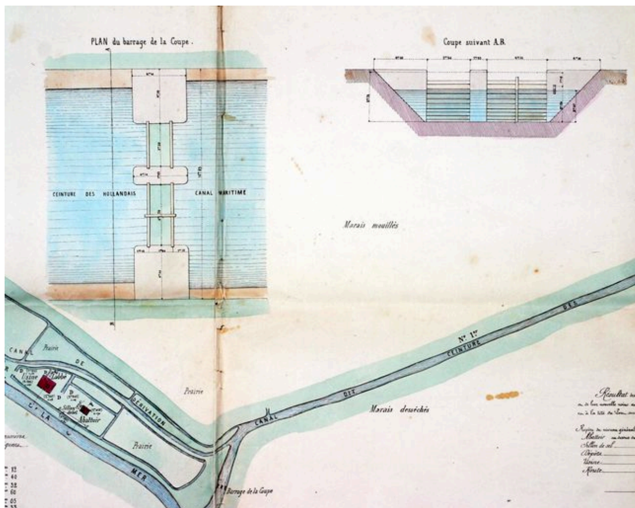
Le barrage de la Coupe (détail d'un plan de Dabin, le 2 juillet 1860).
