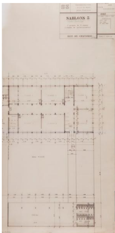
Plan du rez-de-chaussée de l'école Sablons III, juillet 1967. Repro. Pierre-Bernard Fourny IVR52_20197200150NUCA
