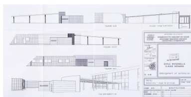
Elévation des façades et du projet de préau arrière pour l'école Gérard-Philipe, 1997. Repro. Pierre-Bernard Fourny IVR52_20197200178NUCA
