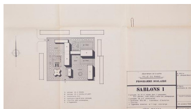
Plan masse de l'école dite Sablons I, 1965. Repro. Pierre-Bernard Fourny IVR52_20197200164NUCA
