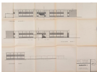
Elévation des façades de l'école Gérard-Philippe, 1965. Repro. Pierre-Bernard Fourny IVR52_20197200166NUCA
