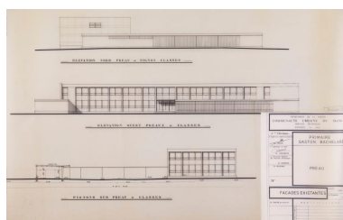
Elévation des façades de l'école Gaston-Bachelard pour la réfection du préau, 1991. Repro. Pierre-Bernard Fourny IVR52_20197200153NUCA
