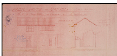
Elévations pour la construction de bureaux au 13 rue Jeanne d' Arc, par l'architecte Victor Rabjeau, pour la SAC, en 1951
