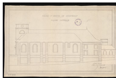
Elévations, 1922.
