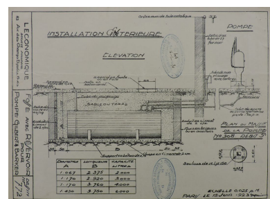
Plan d'installation du réservoir et de la pompe à essence annexé à la demande d'autorisation présentée par Gustave Paré en 1930. Phot. Yannis (reproduction) Suire IVR52_20198503654NUCA
