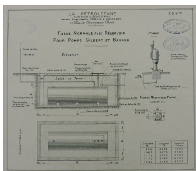
Plan du réservoir et de la pompe à essence, de type Gilbert et Barker, annexé à la demande d'autorisation présentée par Gustave Paré en 1927. Phot. Yannis (reproduction) Suire IVR52_20198503652NUCA
