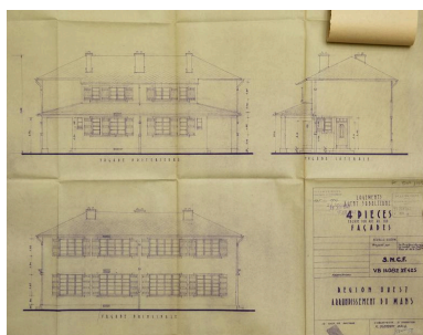
Elévations d'un pavillon double dit Reconstruction, 1947. Repro. Pierre-Bernard Fourny IVR52_20197202606NUCA
