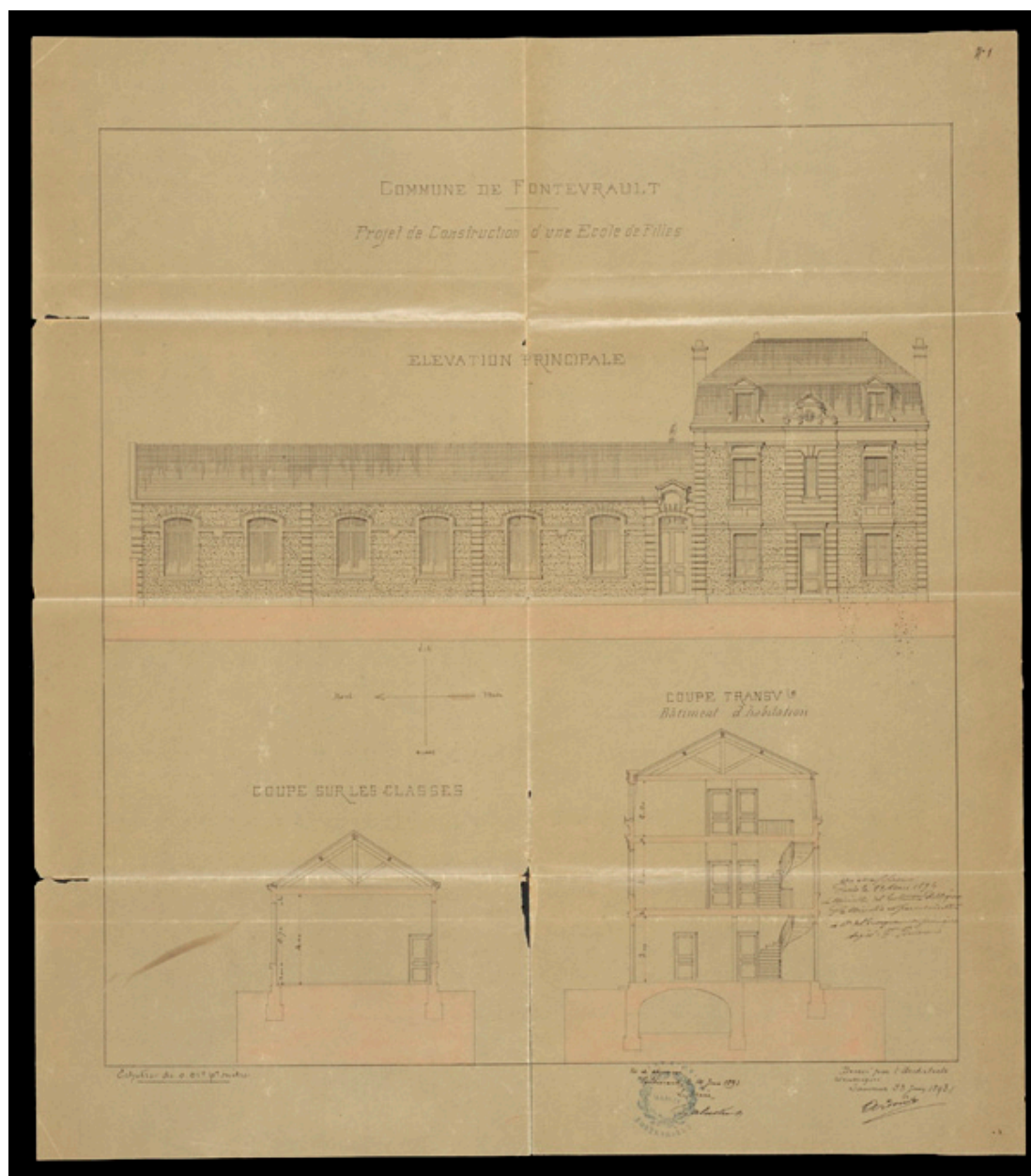
Projet de l'école de filles, en 1893 : élévation et coupes.
