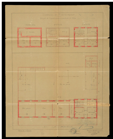
Projet de l'école de filles, en 1893 : plan d'ensemble et plans des niveaux.
