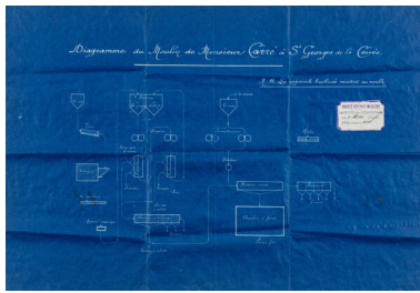
Diagramme schématique du circuit de production, 1907. Repro. Pierre-Bernard Fourny IVR52_20267200021NUCA
