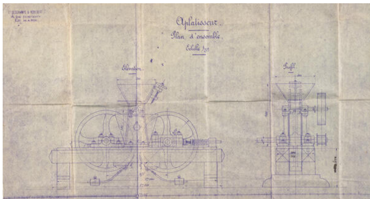
Aplatisseur à grain : plan d'ensemble.
