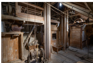
Machines du moulin : comble. Phot. Jeanne Minier IVR52_20257200682NUCA
