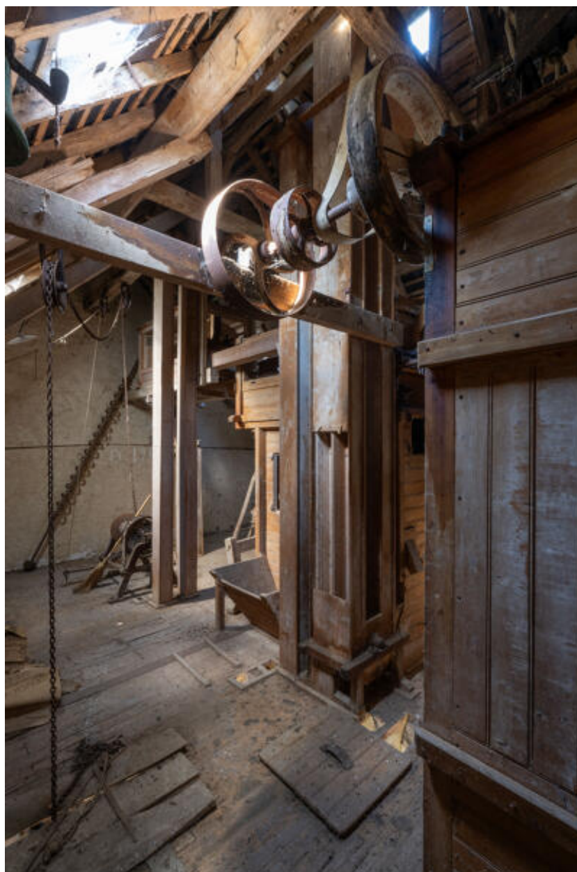
Machines du moulin : comble.
