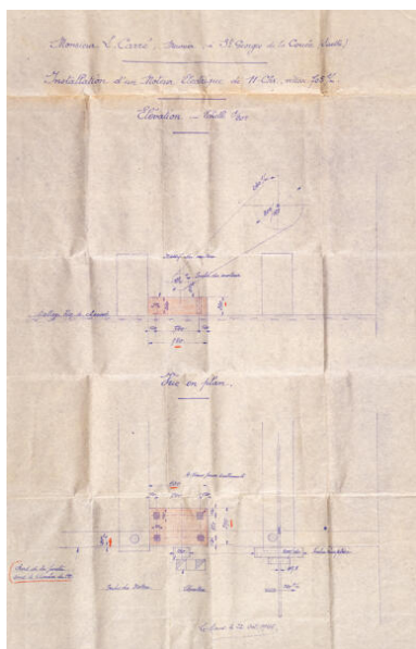
Installation d'un moteur électrique : plan et élévation, 1946. Repro. Pierre-Bernard Fourny IVR52_20267200023NUCA
