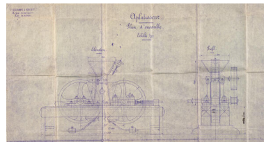
Aplatisseur à grain : plan d'ensemble. Repro. Pierre-Bernard Fourny IVR52_20267200022NUCA
