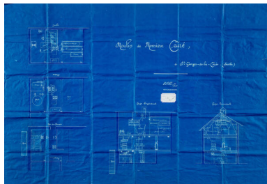
Projet de modernisation avec installation de nouvelles machines : plan et coupes, 1907. Repro. Pierre-Bernard Fourny IVR52_20267200020NUCA
