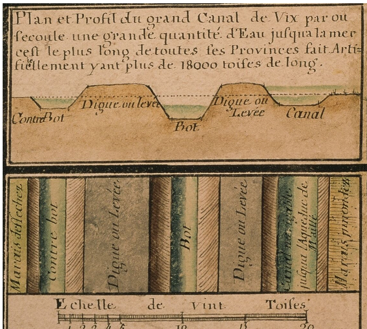
Plan et coupe du canal de Vix, de la Grande levée de Vix et du Contrebote (le canal et le Contrebote sont inversés), par Claude Masse en 1720.
