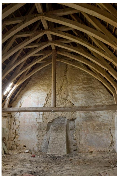
Chapelle : charpente et mur du chœur. Phot. Denis Pillet IVR52_20117200018NUCA
