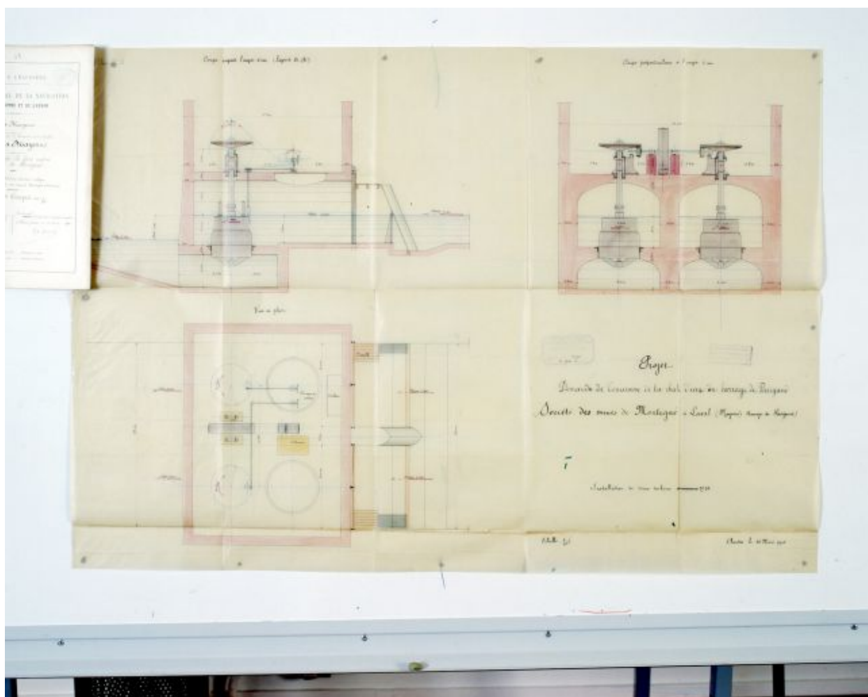
Plan et coupes de l'usine.
