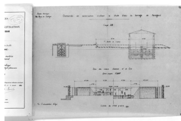
Coupe longitudinale de l'usine et demi-coupes des têtes des canaux d'alimentation et de fuite. Repro. François Lasa
