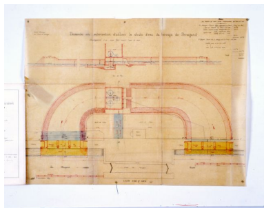
Plan et coupe transversale de l'usine et des canaux d'alimentation et de fuite. Repro. François Lasa
